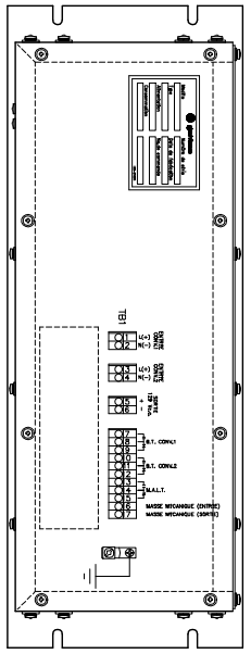
Vue ARRIÈRE
