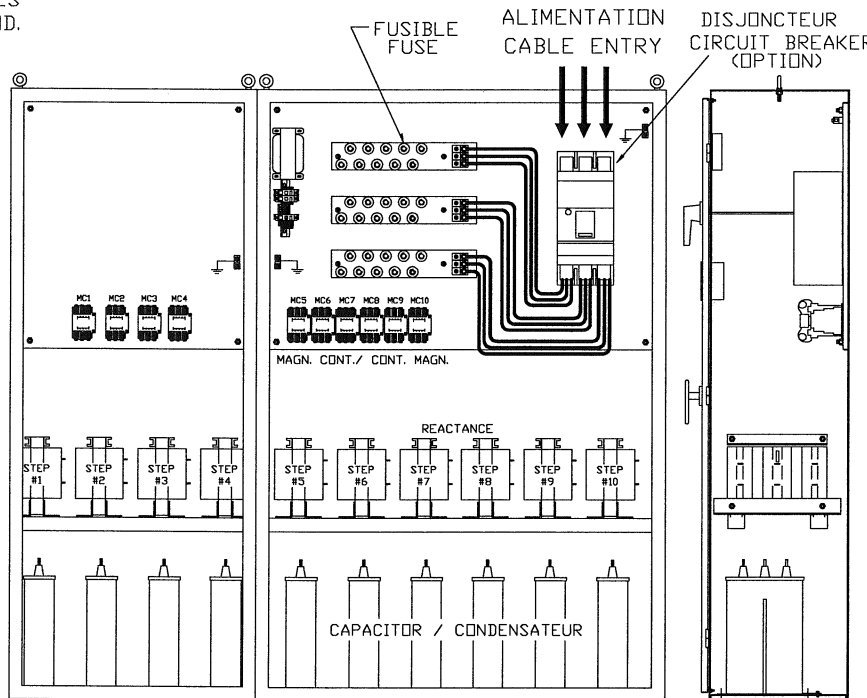
VUE DE COUPE CUT VIEW
