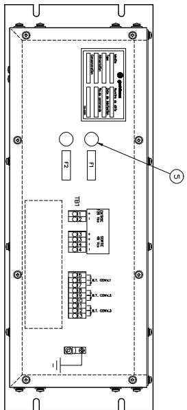
VUE ARRRIERE
